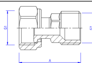
VTr. 613 З'єднувач з накидною гайкою В-3
