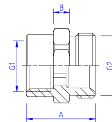
VTr. 592 NE З'єднувач з переходом на «євроконус» В-3
