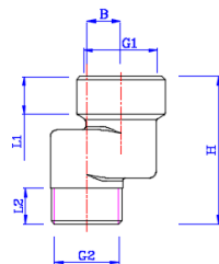
VTр. 094 Ексцентрик В-3
