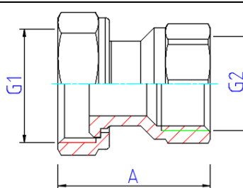
VTr. 614 З'єднувач з накидною гайкою В-В
