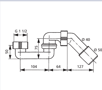
Geruchverschluss für Badewannen Ab- und Überlaufgarnitur aus Kunststoff, mit Ablaufbogen Ø 40/50 mm, Verpackung im Foliebeutel
