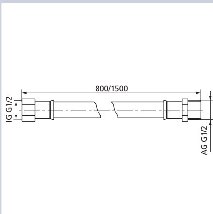
Anschlusschlauch mit Nippel, 1/2" Außengewinde, 1/2" Überwurfmutter mit Dichtung, Verpackung im Foliebeutel
