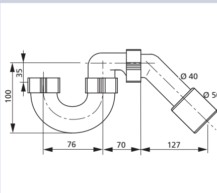
Rohrgeruchverschluss für Badewannen Ab- und Überlaufgarnitur aus Kunststoff, mit Ablaufbogen Ø 40/50 mm, Verpackung im Foliebeutel
