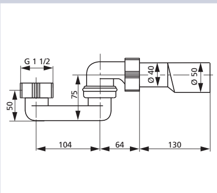
Geruchverschluss für Badewannen Ab- und Überlaufgarnitur aus Kunststoff, Ablauf waagrecht Ø 40/50 mm, Verpackung im Foliebeutel
