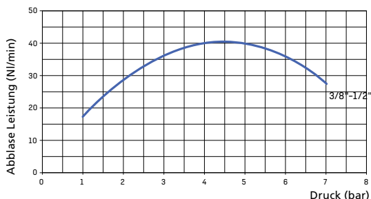
DIAGRAMM DER BETRIEB DES SCHNELLENTLÜFTER MIT SEITENABLAUF
