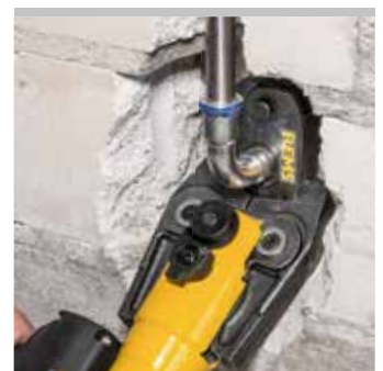
Пресс-кольца REMS 45° (PR-2B) Патент EP 2 774 725
