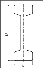
ПРОФИЛЬ АЛЮМИНИЕВЫХ РЕШЕТОК
