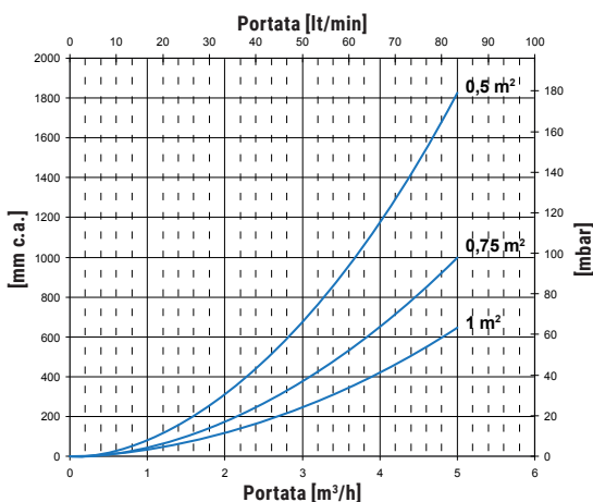
Grafico per superfici: 0,5 m 2 / 0,75 m 2 / 1 m 2
