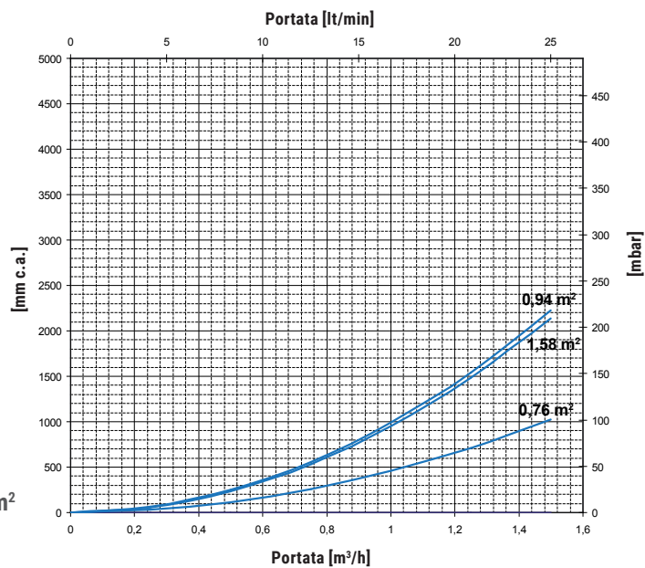
Superfici scambiatori
