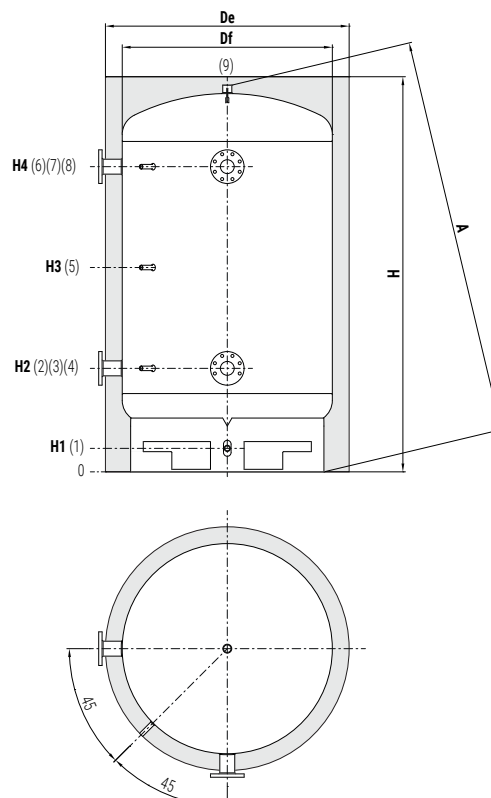
CONNESSIONI FLANGIATE A 90°
