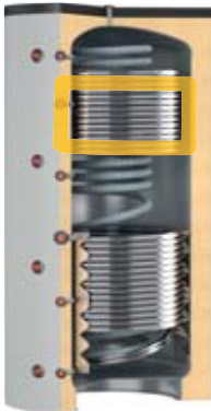
Superfici scambiatori superiori
