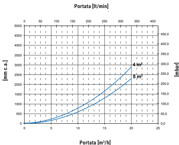
Grafico per superfici: 4 m 2 / 5 m 2
